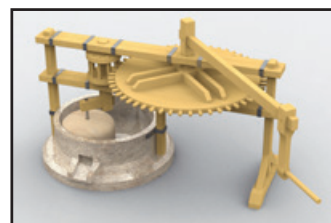
ręczny młyn
